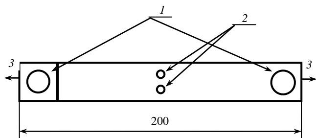
Рис. 3. Схема образца, испытываемого по методу исследования горячей пластичности: 1 — усилители; 2 — концентраторы напряжения; 3 — направление усилия разрыва
